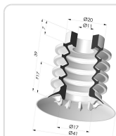
Ventosa 4.5 Fole Série 95 Ø 41MM
