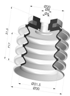
Ventosa 4.5 Soffietti Serie 92 Ø 30MM
