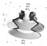
Ventosa 1.5 Soffietti Serie 91 Ø 50MM Riferimento prodotto: 91 50-- A
