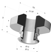
Inserto a resca Femmina G1/8" Riferimento prodotto: 9G18-2
