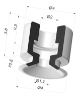
Ventosa Piatta PFG Ø 4 mm
