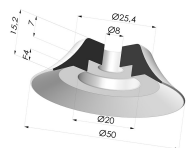
Ventosa Piatta Serie PFG Ø 50 mm
