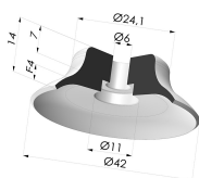
Ventosa Piatta Serie PFG Ø 42 mm
