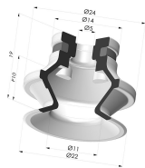
Ventosa 1.5 Soffietti Serie 91 Ø 22,2MM Riferimento prodotto: 91 20-- A
