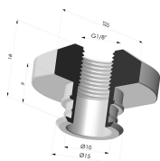
Inserto a resca Femmina G1/8"
