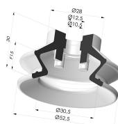
Ventosa 1.5 Soffietti Serie 97B Ø 52.5MM
