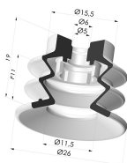
Ventosa 2.5 Soffietti Serie 96C Ø 25MM
