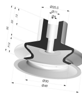
Ventosa 1.5 Soffietti Serie 8A Ø 49MM
