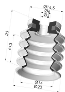
Ventosa 4.5 Soffietti Serie 92 Ø 20MM
