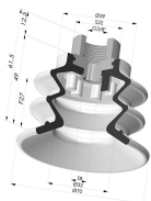
Ventosa 2.5 Soffietti Serie 96C Ø 70MM
