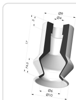
Ventouse 1.5 Soufflets Série 91 Ø 10,2MM Référence produit : 91 11-- A
