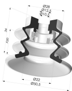
Ventosa 2.5 Fuelles Serie 96C Ø 50MM
